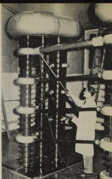
El generador de alta tensión para el acelerador Cockcroft-Walton
