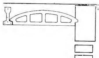
A.—Detalle de bovedilla y su montaje.
